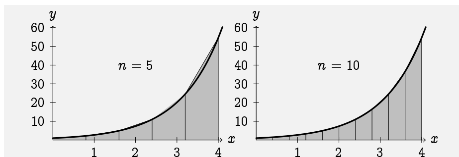
Figura 1.27: Aproximaciones usando n = 5 y n = 10 .
