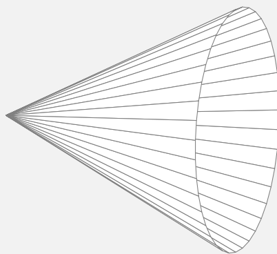
Figura 1.20: Cono de revolución resultante.
