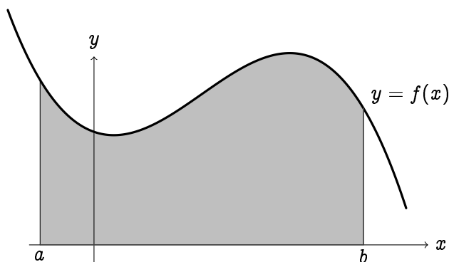
Figura 1.1: Área bajo una curva.
