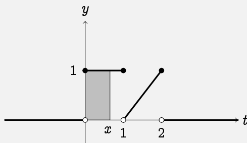
Figura 1.5: Función integral para 0 \leq x \leq 1
