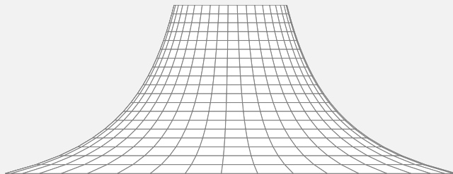
Figura 1.22: Sólido de revolución resultante.
