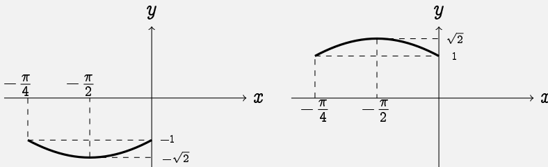
Figura 4.4: Gráfico de una función y su módulo.
