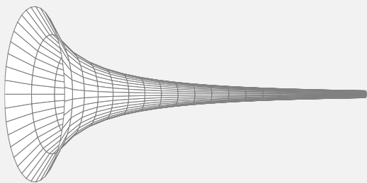
Figura 1.23: Trompeta de Torricelli.
