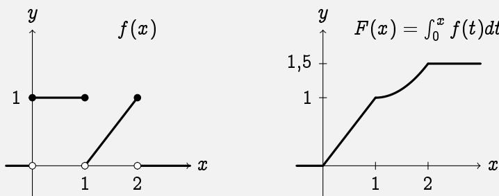
Figura 1.7: Función f y su función integral.
