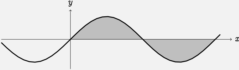
Figura 1.11: Región encerrada por el gráfico de f(x) = \operatorname{sen}(x) y el eje x para 0 \leq x \leq 2\pi .
