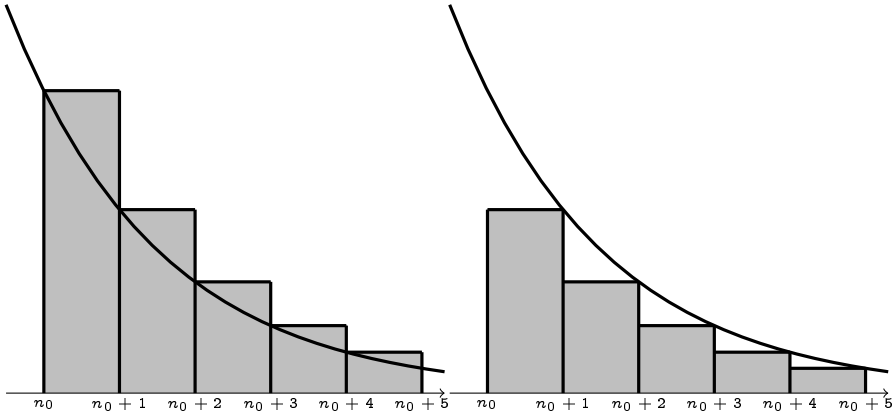
Figura 5.2: Criterio Integral de Cauchy.
