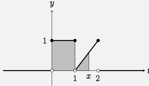
Figura 1.6: Función integral para 1 < x \leq 2 .
