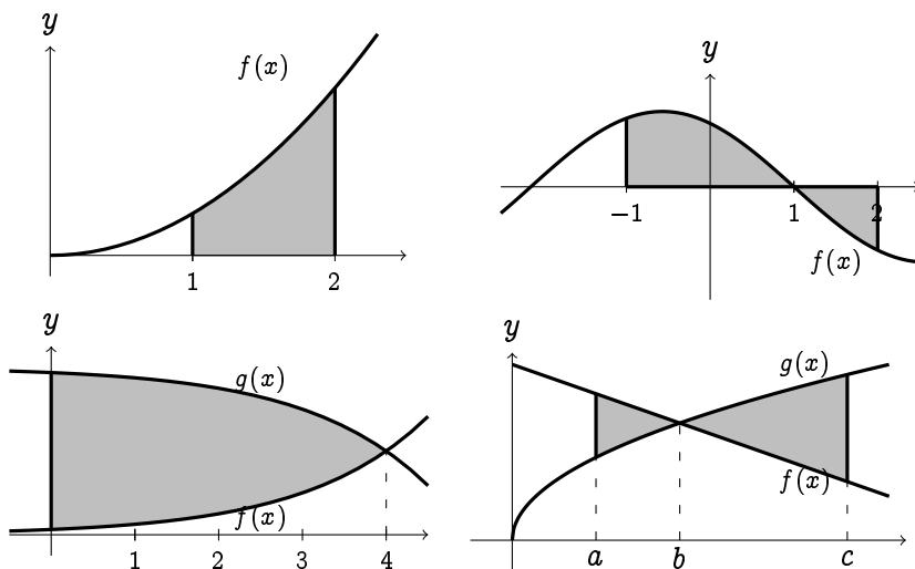
Figura 1.24: Áreas.
