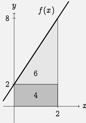
Figura 1.4: El área debajo de f se descompone en un cuadrado y un triángulo.
