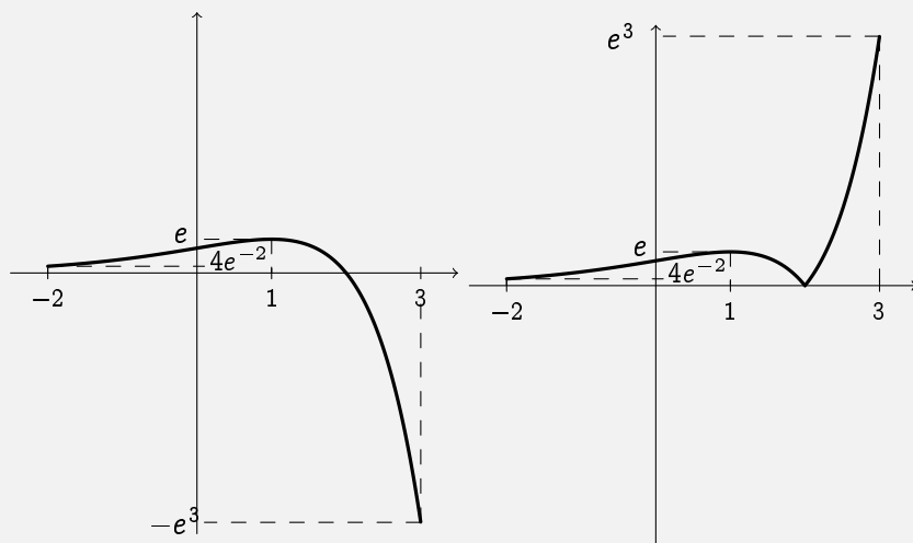
Figura 4.3: Ejemplo 4.2.3.
