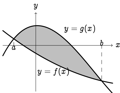
Figura 1.12: La región S encerrada entre dos curvas.
