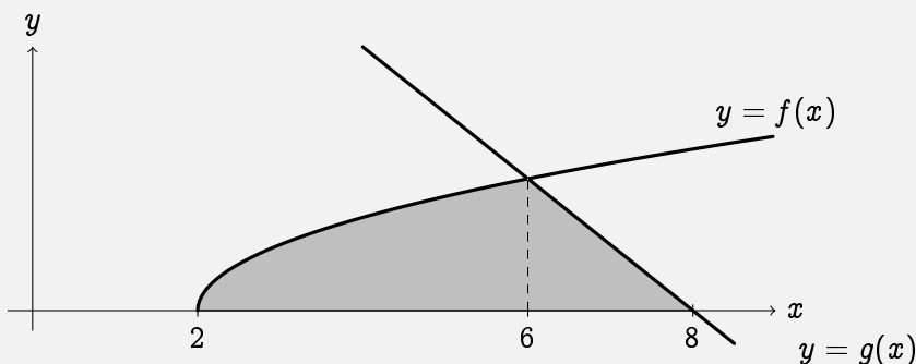
Figura 1.17: Área encerrada entre el gráfico de f , el de g y el eje x .
