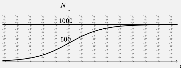
Figura 2.1: Campo de direcciones la ecuación diferencial.
